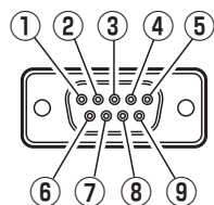
(背面側から見たピン配置図)
